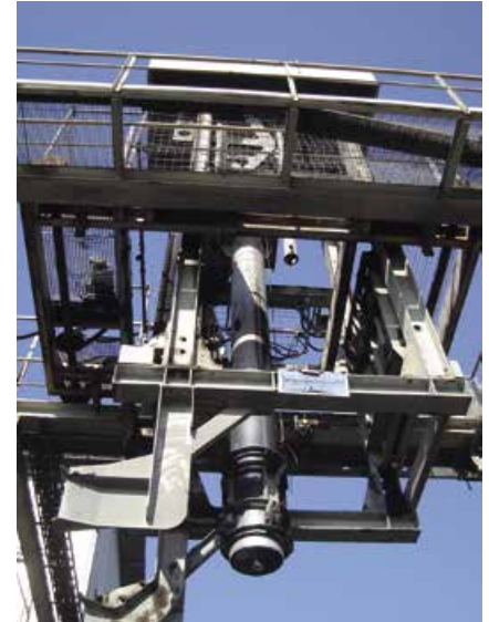
Probenehmer bestehend aus Bohrschnecke mit Säuberungsschaber, Fahrwerk und Hubwerk
