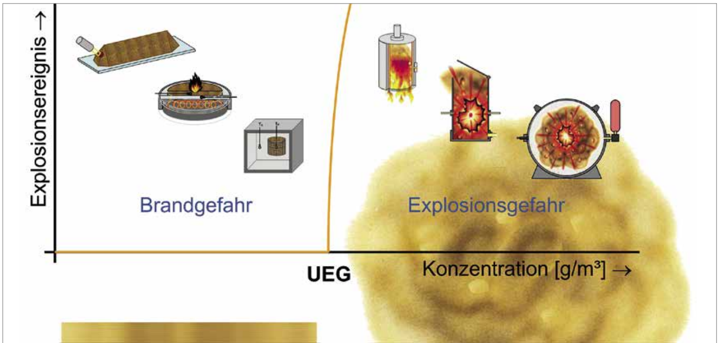
Bild 2: Untere Explosionsgrenze, Abgrenzung Brand- und Explosionsgefahr
