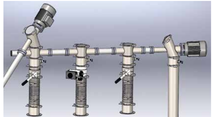
Die Mehrstellenbeschickungsanlage Typ PM eignet sich zur Beschickung einer Reihe von Maschinen
